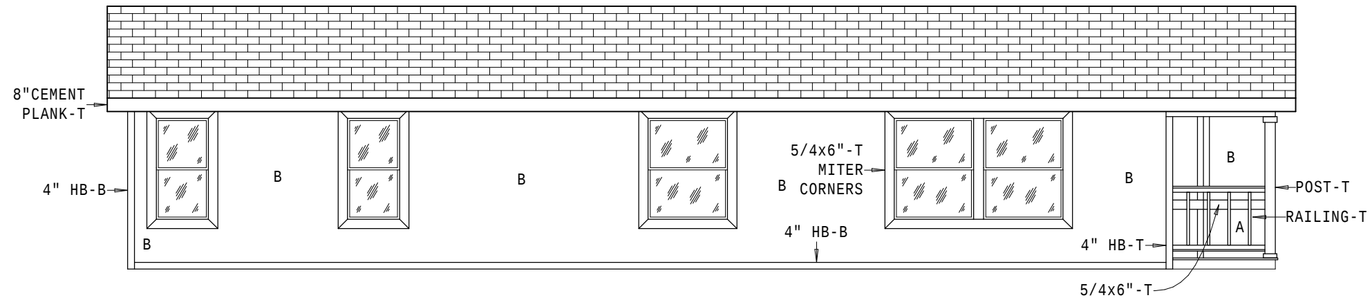
DOOR SIDE ELEVATION
